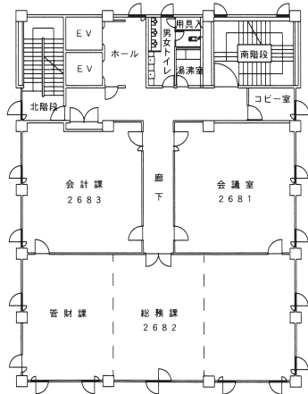
8階 平面図
