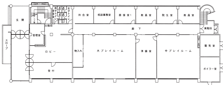
1階 平面図
