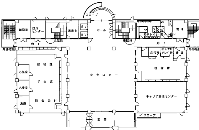
1階 平面図
