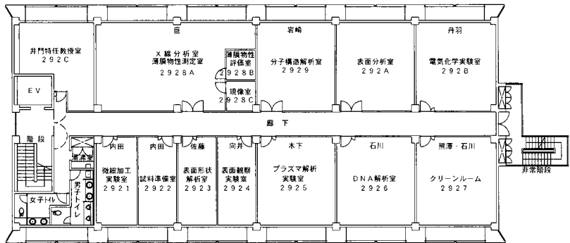
2階 平面図
