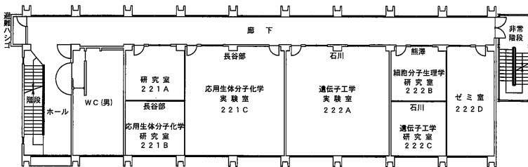
2階 平面図
