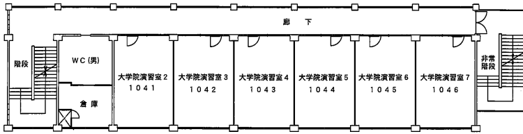
4階 平面図
