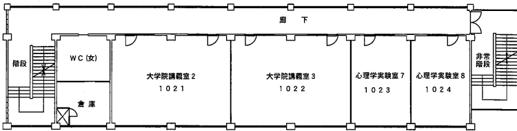
2階 平面図
