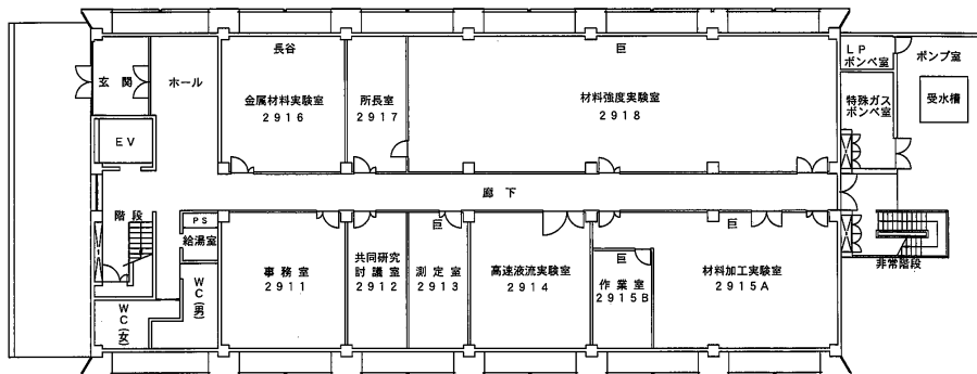
1階 平面図
