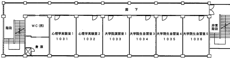
3階 平面図
