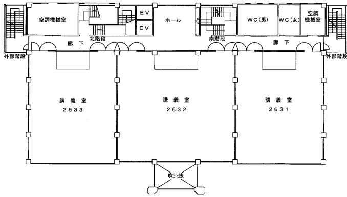
3階 平面図
