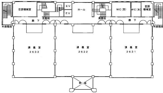
3階 平面図
