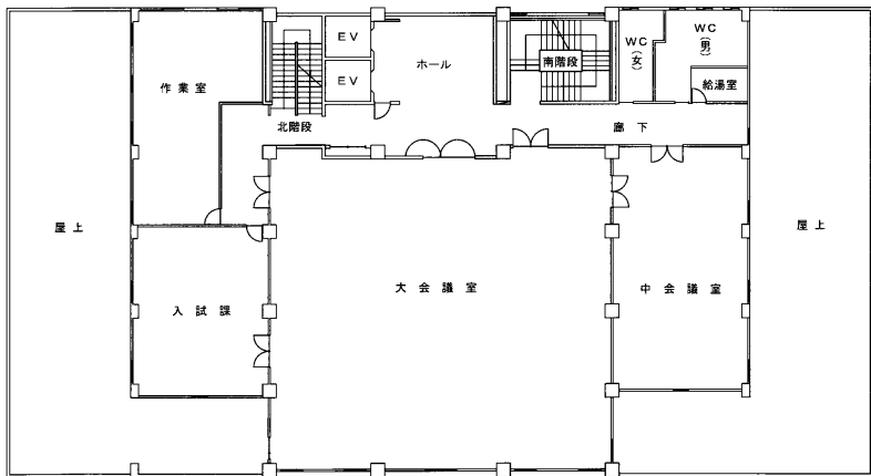
4階 平面図
