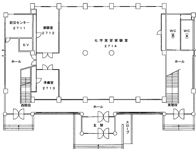
1階 平面図
