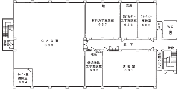
3階 平面図
