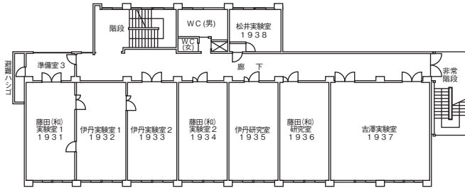
3階 平面図
