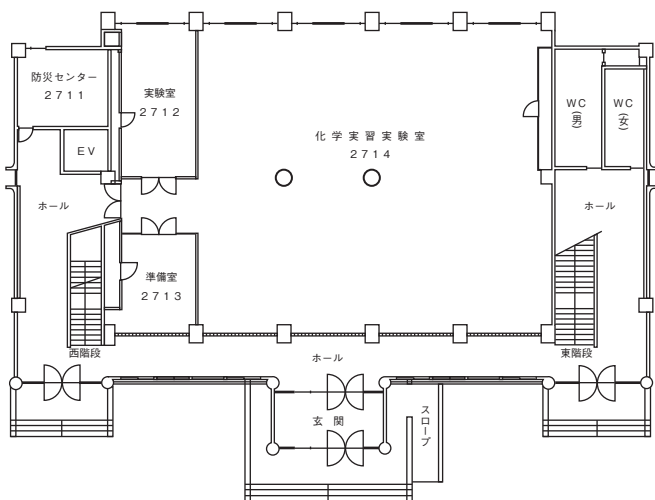
1階 平面図
