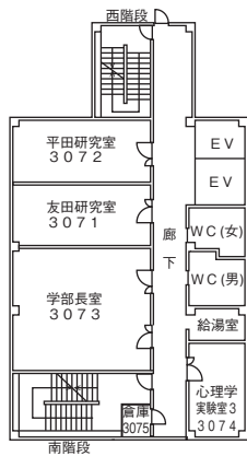
7 階 平面図
