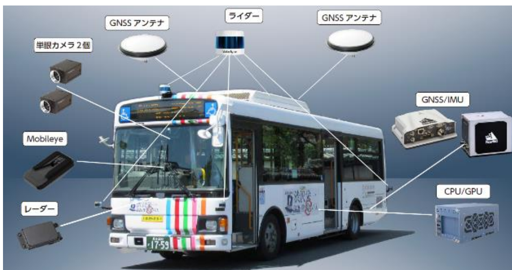
《埼玉工業大学の自動運転バス》
