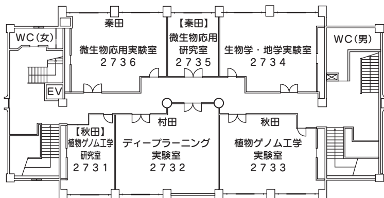
3階 平面図
