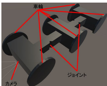
図1:Blender により作成したヘビ型災害ロボット
