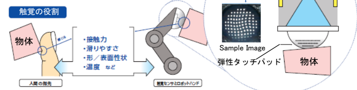
図2 触覚センサ
