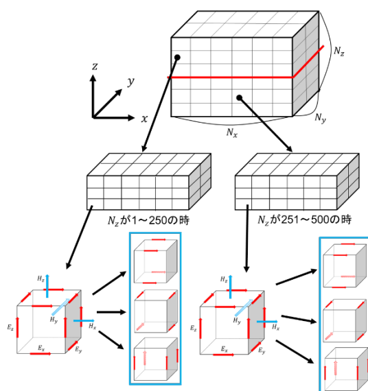
図1 三次元電磁界計算の並列化技術 1)
