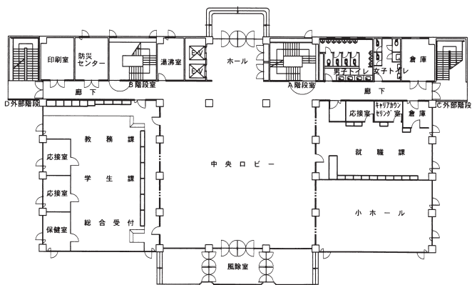
1 階 平面図
