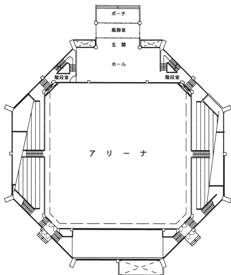
1階 平面図
