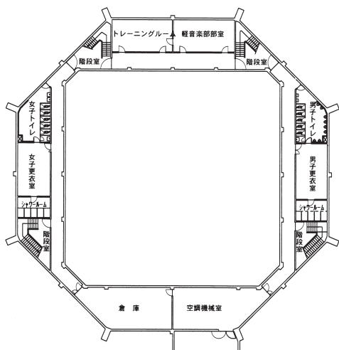
地階 平面図
