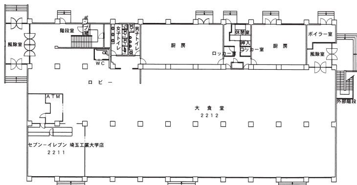
1階 平面図
