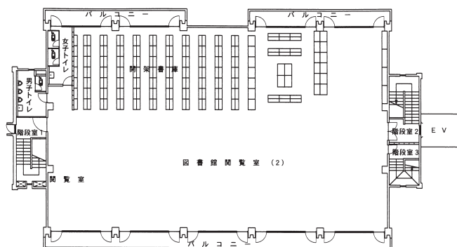
3階 平面図
