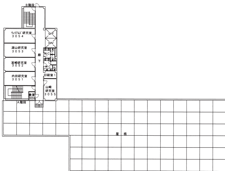
5 階 平面図
