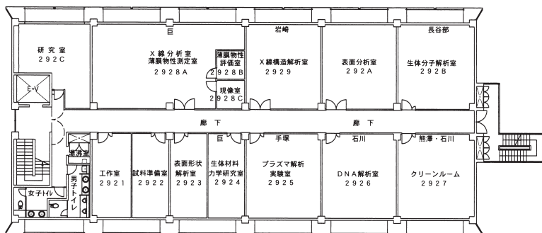
2階 平面図
