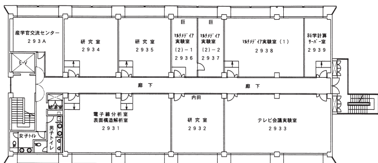
3階 平面図
