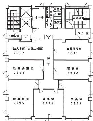
9階 平面図
