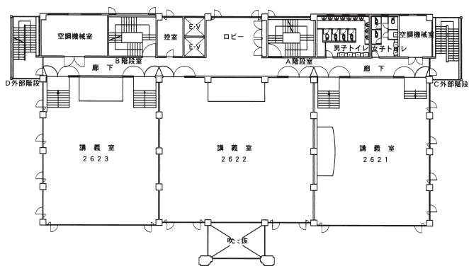
2 階 平面図
