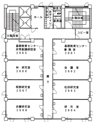
6階 平面図
