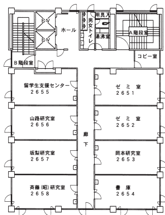
5階 平面図
