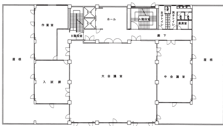
4階 平面図
