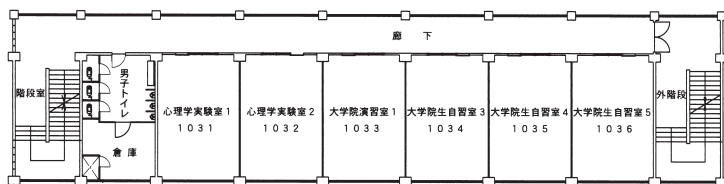
3 階 平面図
