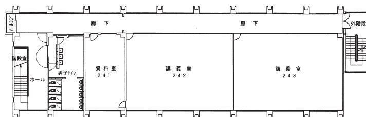
4階 平面図
