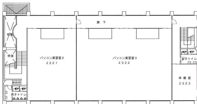
2階 平面図
