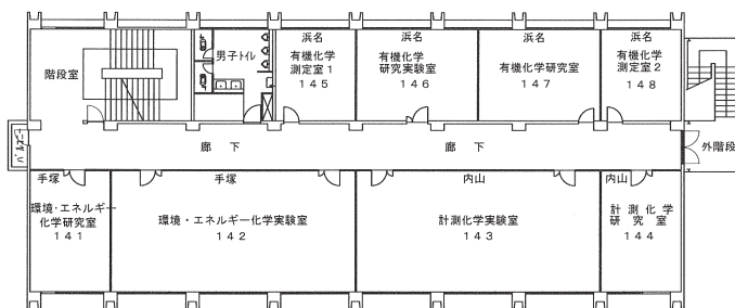
4 階 平面図
