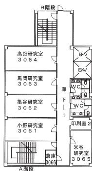
6階 平面図
