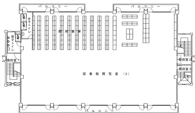
3階 平面図
