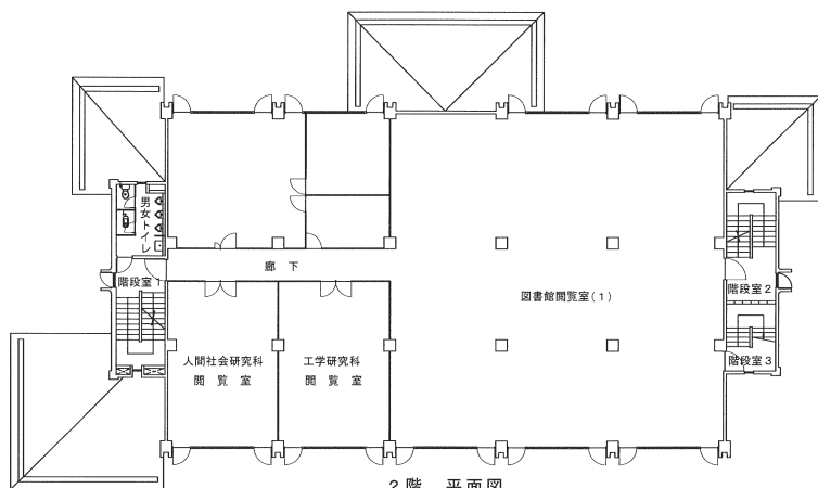
2階 平面図
