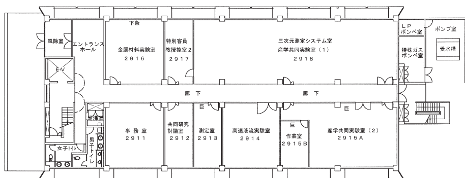
1階 平面図
