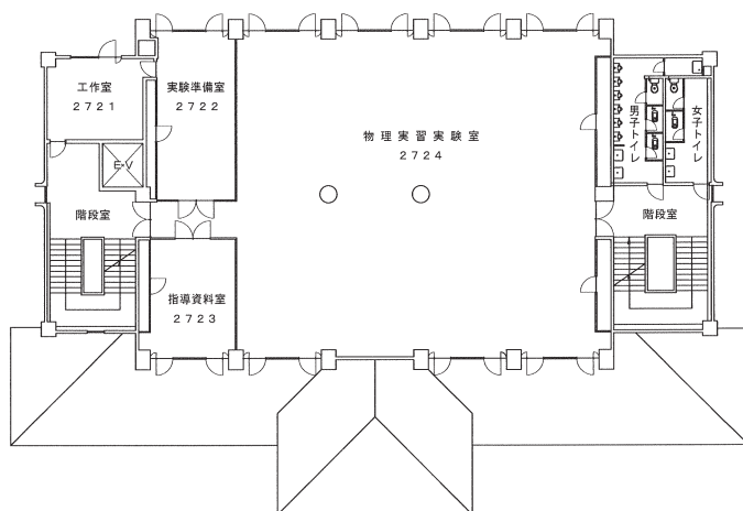
2階 平面図
