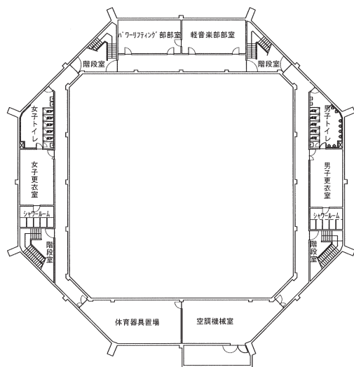
地階 平面図
