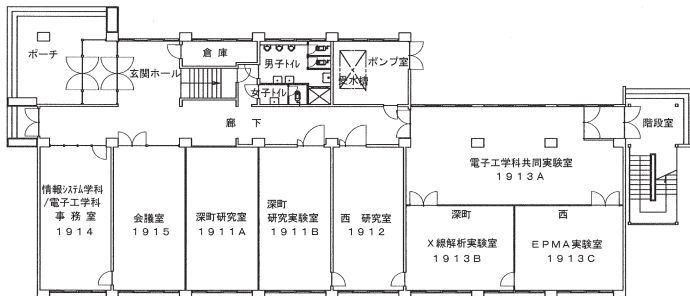
1階 平面図
