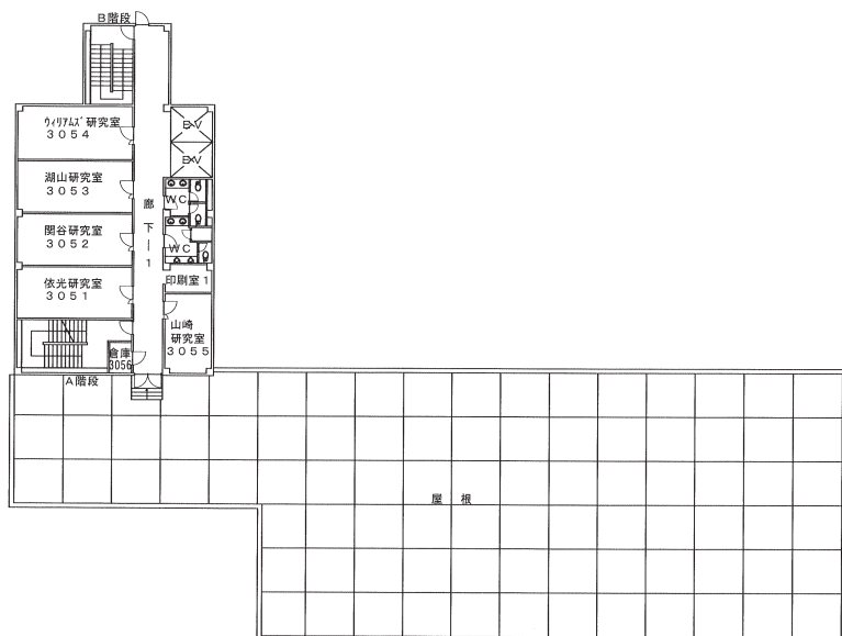
5階 平面図
