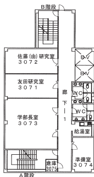
7階 平面図
