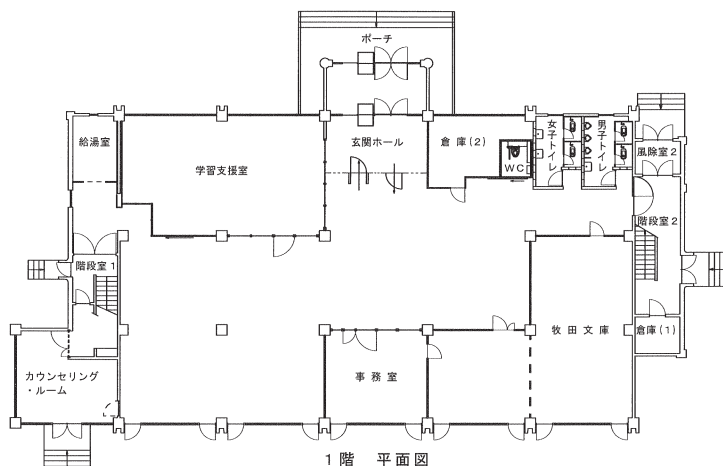
1階 平面図
