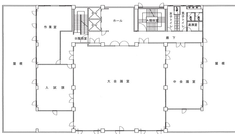
4階 平面図
