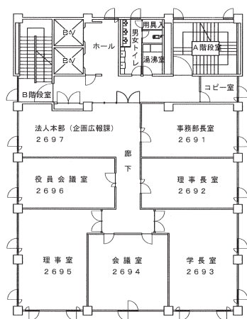
9階 平面図
