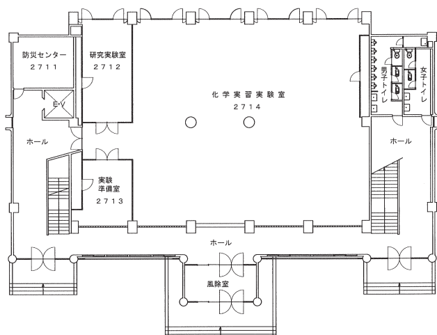
1階 平面図
