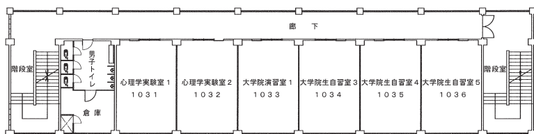
3 階 平面図
