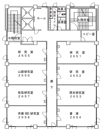
5階 平面図
