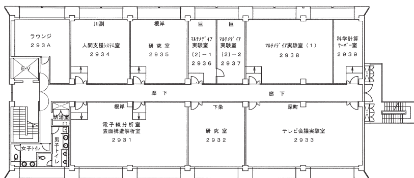
3階 平面図
